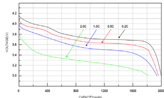
图 2: 2000mAh 锂离子电池的典型放电曲线
