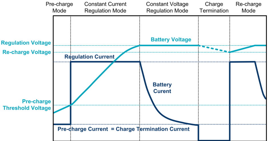
图 3：锂离子电池充电模式
